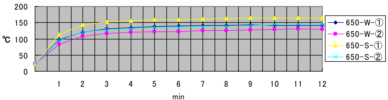
塗板温度上昇データ（JCD120V-650Wタイプ） 塗板①グレー 塗板②クリーム 距離250mm
